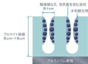
アルマイトイメージ図
