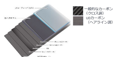
勝色カーボン模式図
