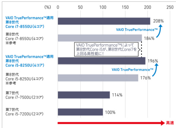
従来プロセッサーとのパフォーマンス比較 CPU: MAXON Cinebench Version 15.0.3.8 でのベンチマークスコア
