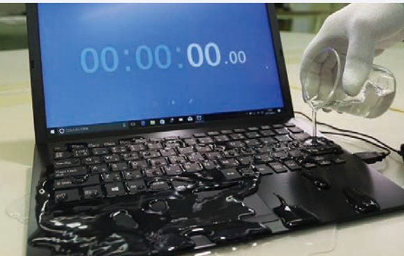
キーボード水かけ試験 (VAIO Pro PJ / PG / PK / PA で実施)
